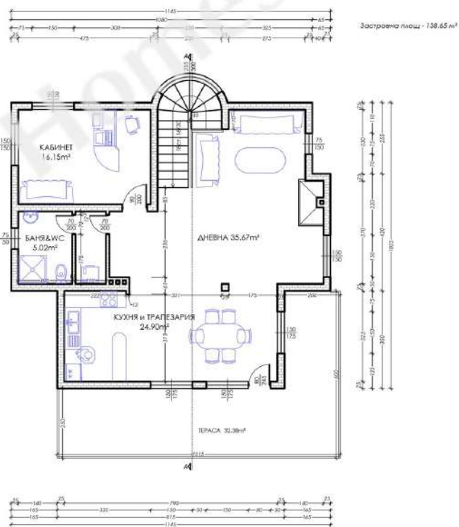
ТРЕТИ ЕТАЖ/ THIRD FLOOR
