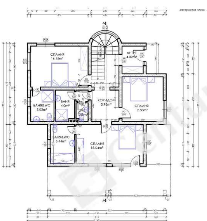
ВТОРИ ЕТАЖ/ SECOND FLOOR
